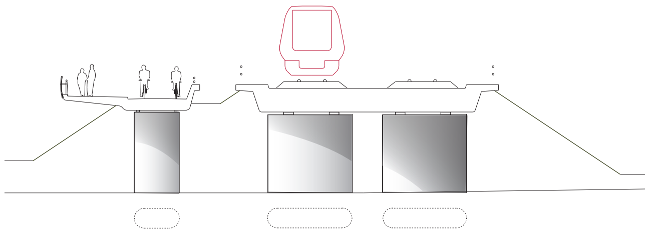
Gang- og cykelbro og banebro for Ringbanen, 1:200
