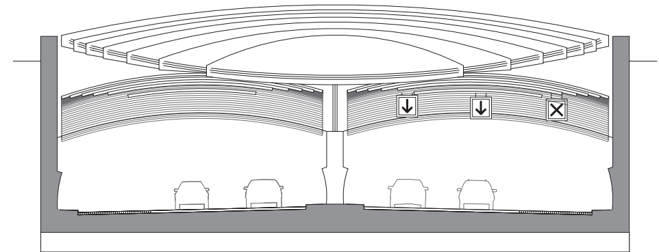
Snit B 1:200
