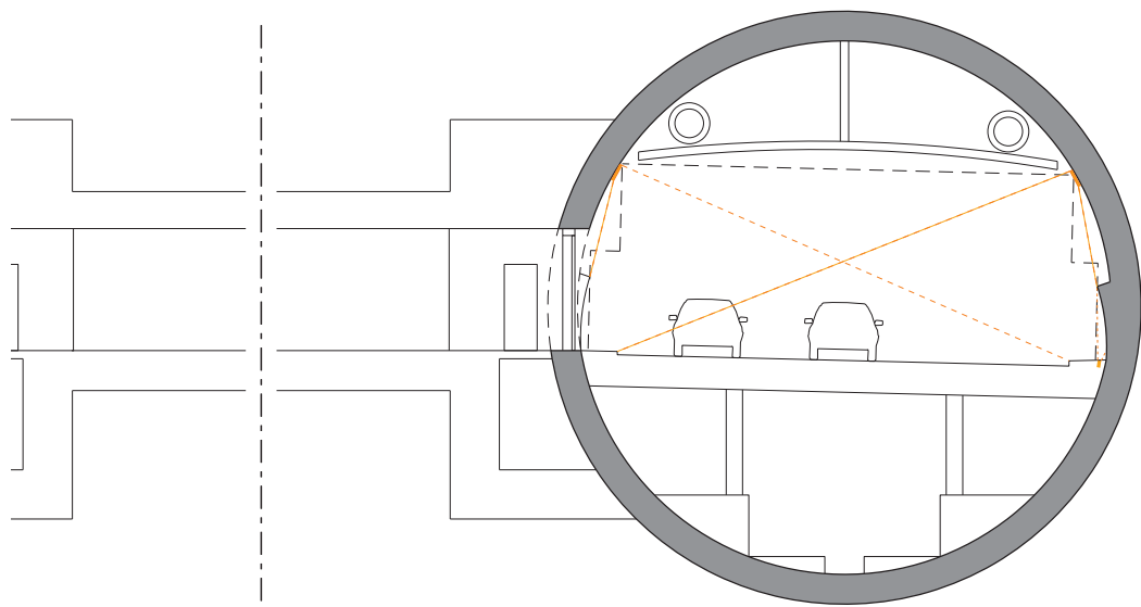
snit D 1:200
