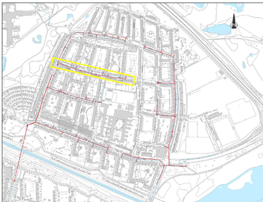
Figur 1: Kort over Tingbjerg. Ledningsplacering markeret med rødt. Vegen Arkaderne (gul firkant), hvor regn- og spildevandsledninger anlægges ved pilotrørsmetoden.
