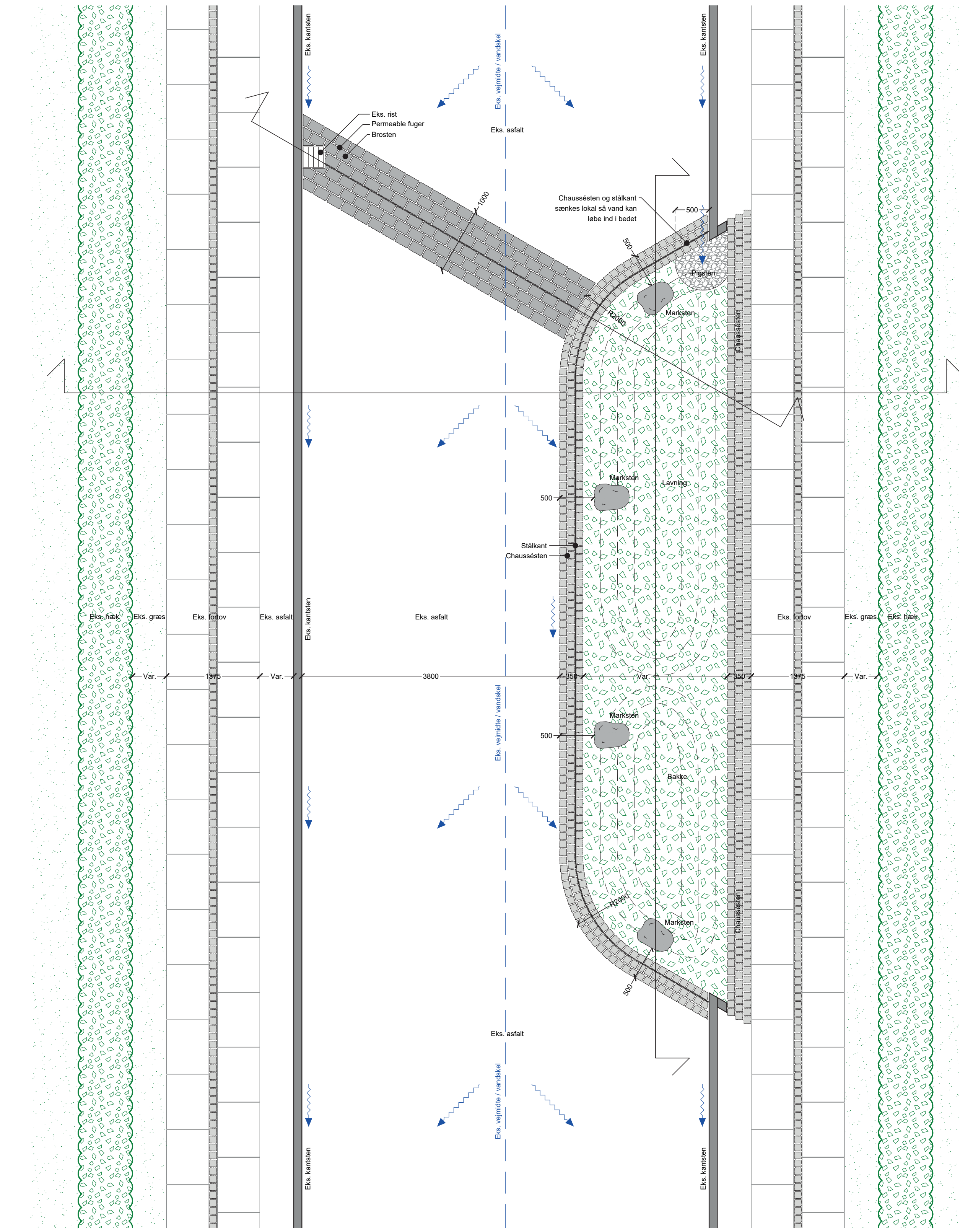
PLAN 1:50
