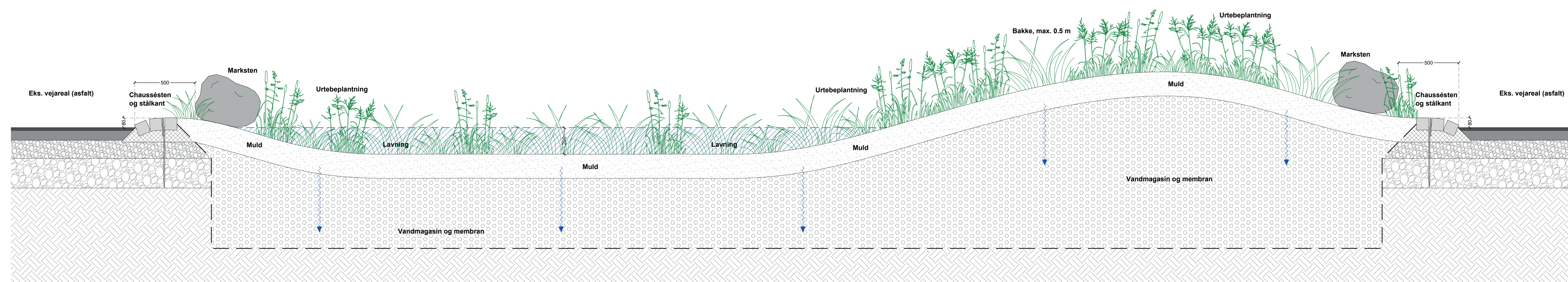
LÆNGDESNI 1:20
