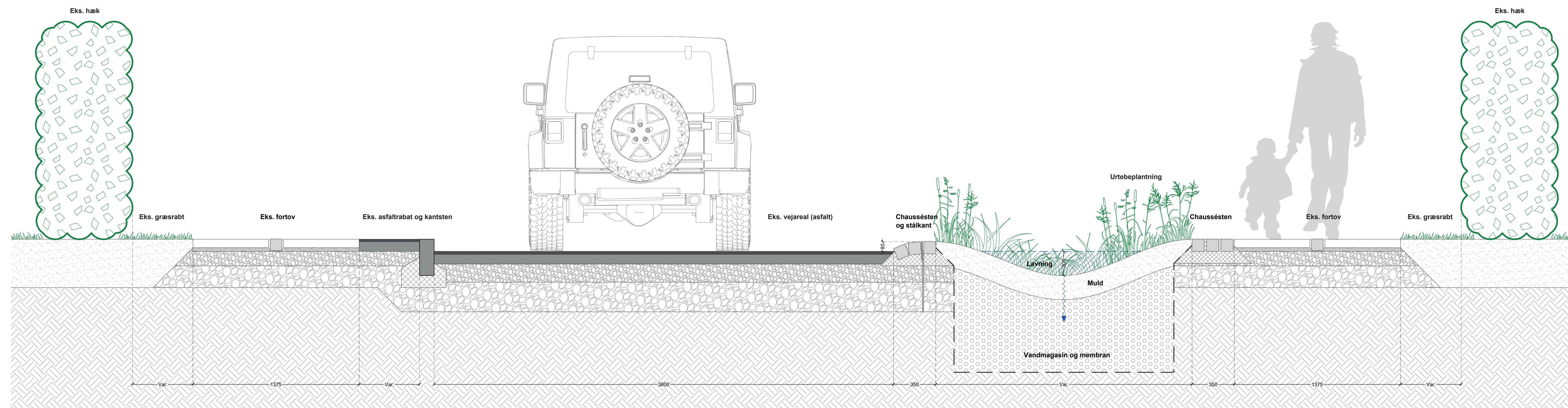
TVÆRSNIT 1:20
