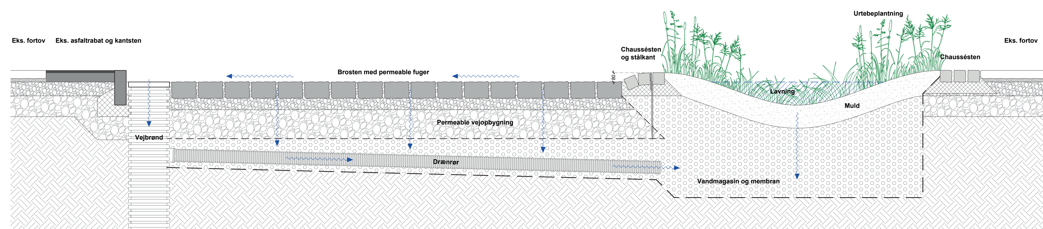
TVÆRSNIT | CROSSING 1:20
