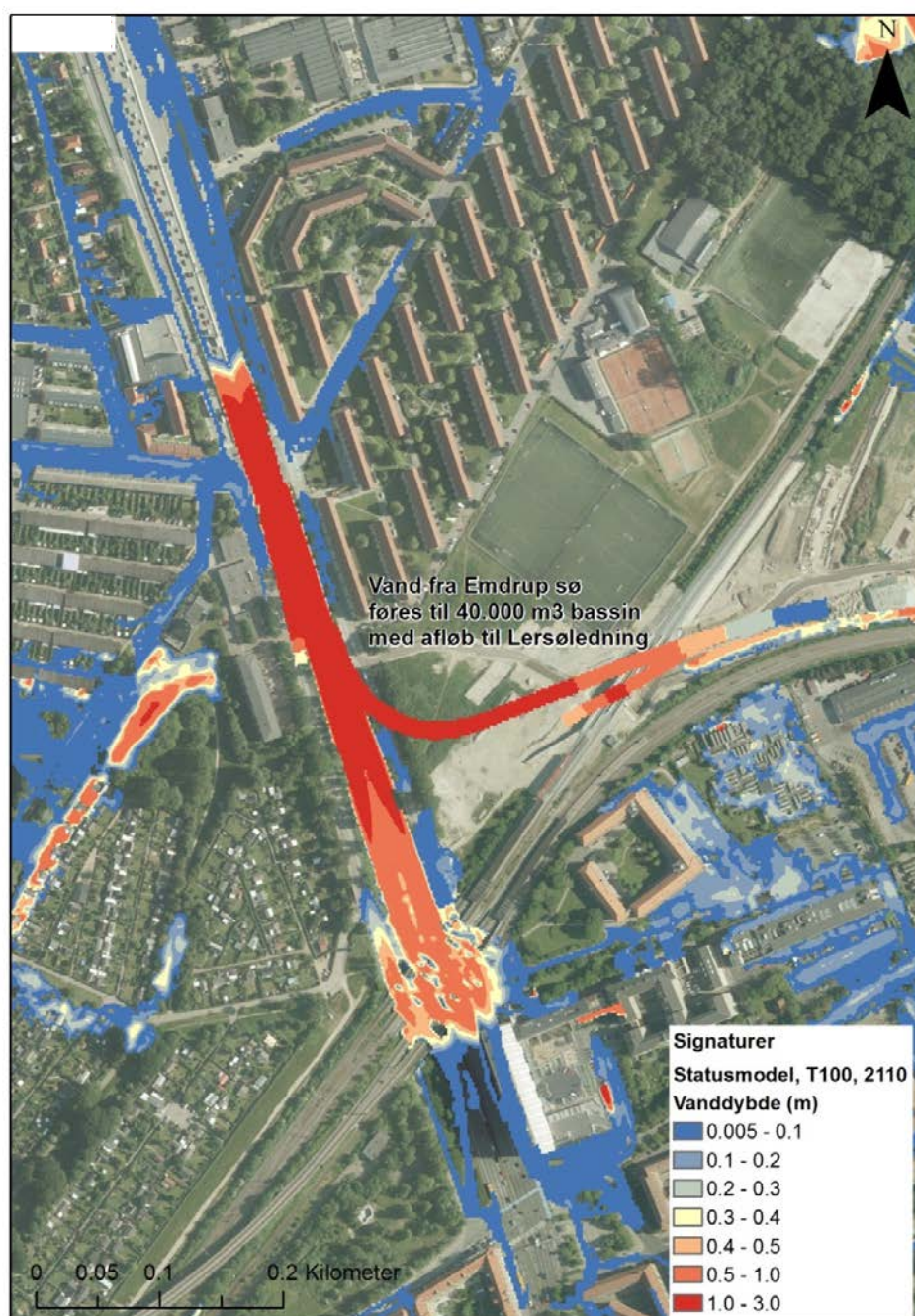
Figur 5-18 Oversvømmelser ved Lyngbyvej/Helsingørmotorvejen før tiltag for 100 års regnhændelse i 2110.
