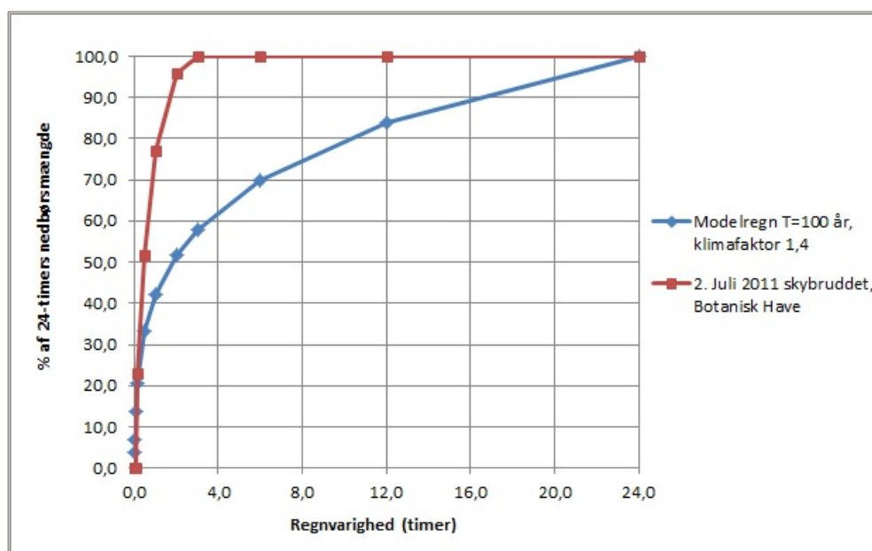
Figur 3-4 Procentvis fordeling af 24-timers nedbørsmængden for 2. juli 2011 skybruddet i Botanisk Have og 100-års modelregnen.
