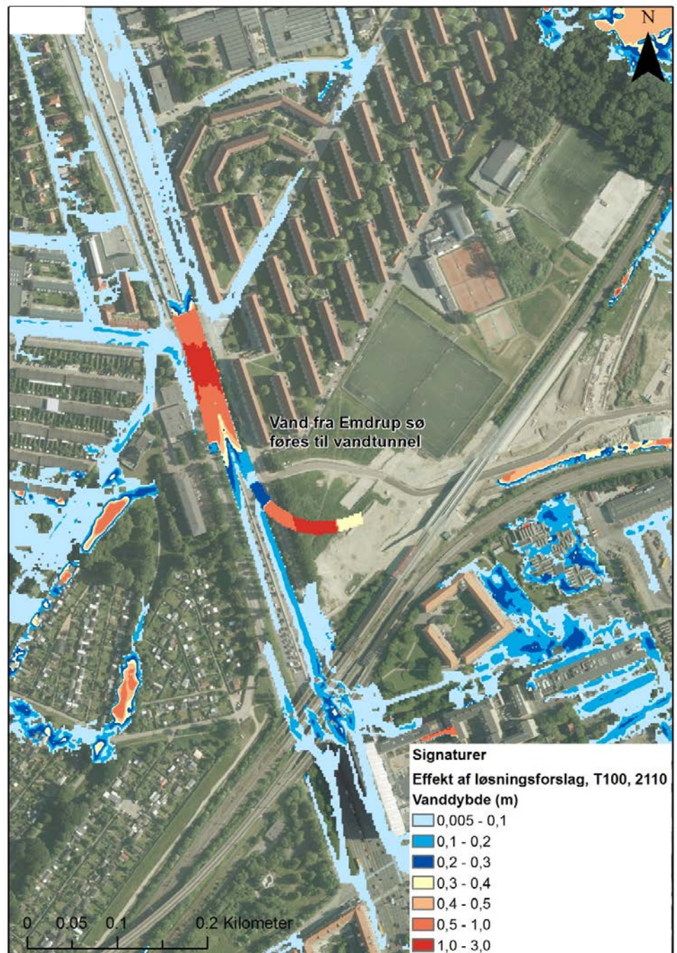
Figur 5-19 Oversvømmelser ved Lyngbyvej/Helsingørsmotorvejen efter tiltag for 100 års regnhændelse i 2110. Grunden til oversvømmelserne er at Lyngbyvejs, Helsingørsmotorvejens og Nordhavnsvejs afvandingsystemer er dimensionerede til mindre end 100 års regnhændelse.
