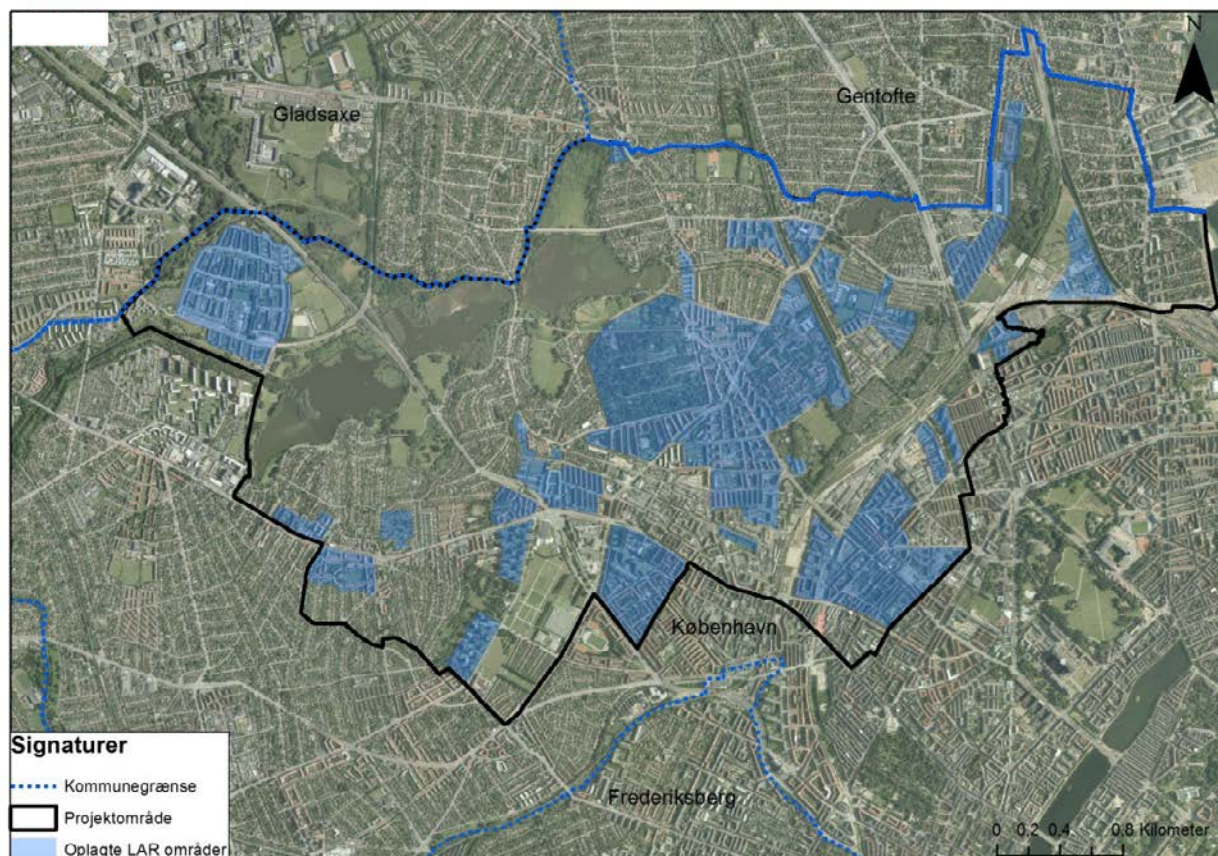
Figur 5-41 Områder i projektområdet, hvori det vil være oplagt at afkoble regnvand med LAR. På lokaliteter med kortlagte jordforureninger vil nedsivning dog ikke kunne tillades – se Figur 5-38.
