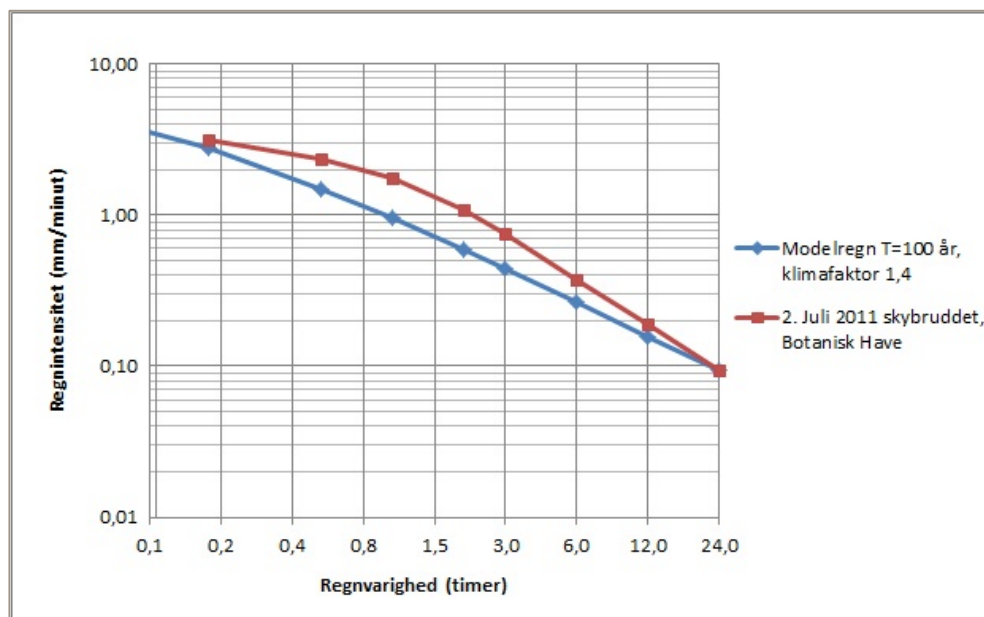
Figur 3-3 Regnkurver for 2. juli 2011 skybruddet baseret på aflæsning i Figur 3-1 af de 3 højeste radarberegnete intensiteter for pixels omkring Botanisk Have og 100-års modelregnen.
