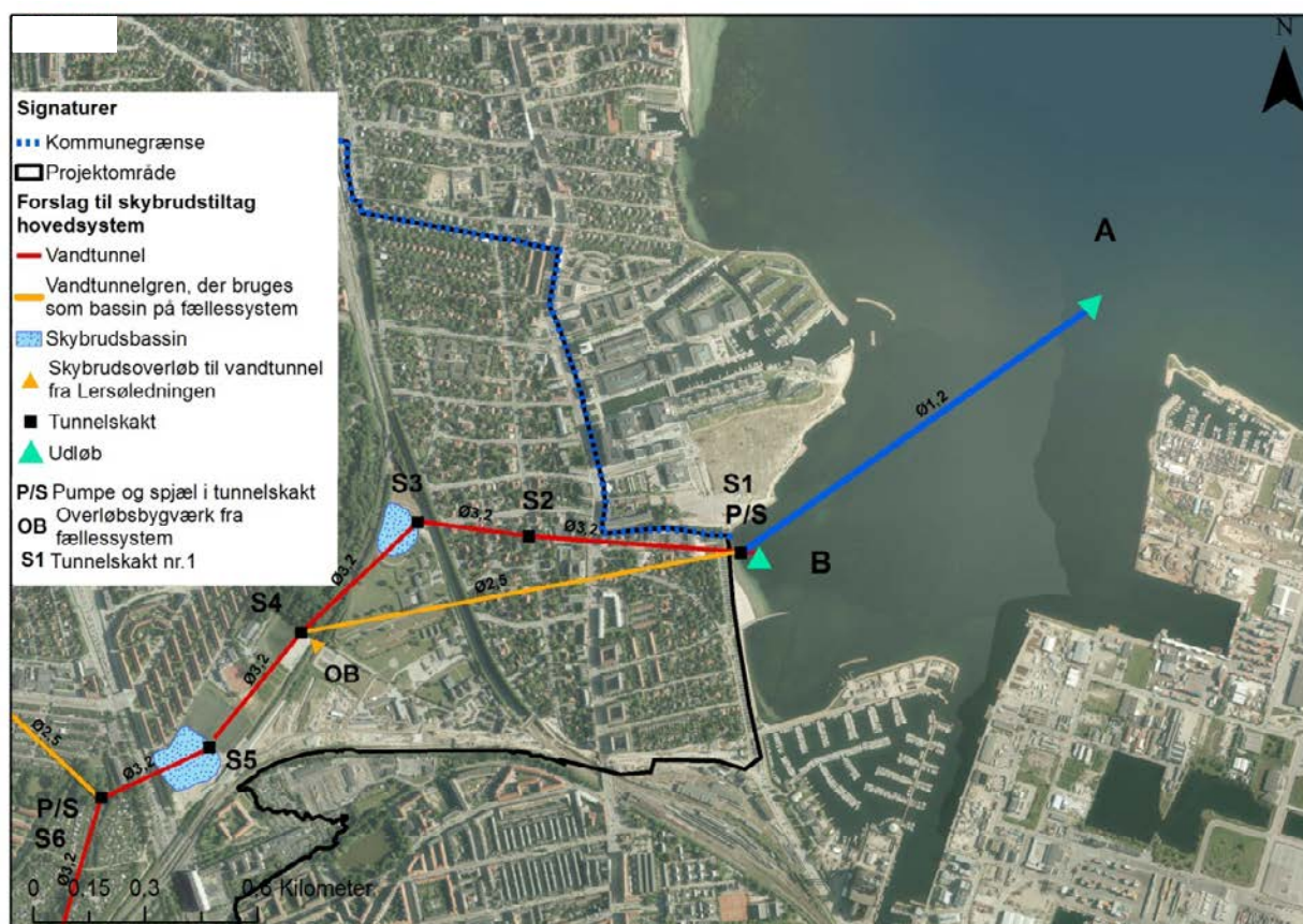
Figur 5-17 Nye Udløb A og B fra vandtunnel i Svanemøllebugten. Alternativ placering af vandtunnelens udløbsarrangement i Københavns Kommune.
