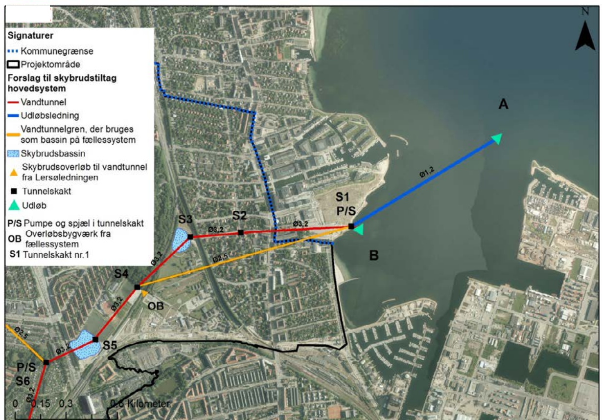
Figur 5-16 Nye Udløb A og B fra vandtunnel i Svanemøllebugten. Vandtunnelens udløbsarrangement er placeret i Gentofte Kommune på Tuborg Syd.
