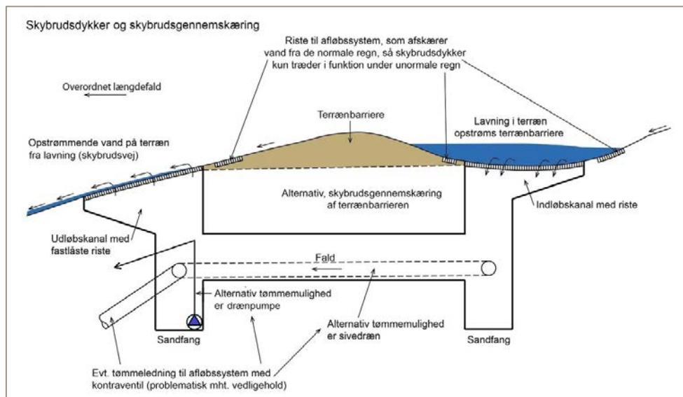
Figur 5-32 Princip i skybrudsgennemskæring og skybrudsdykker.
