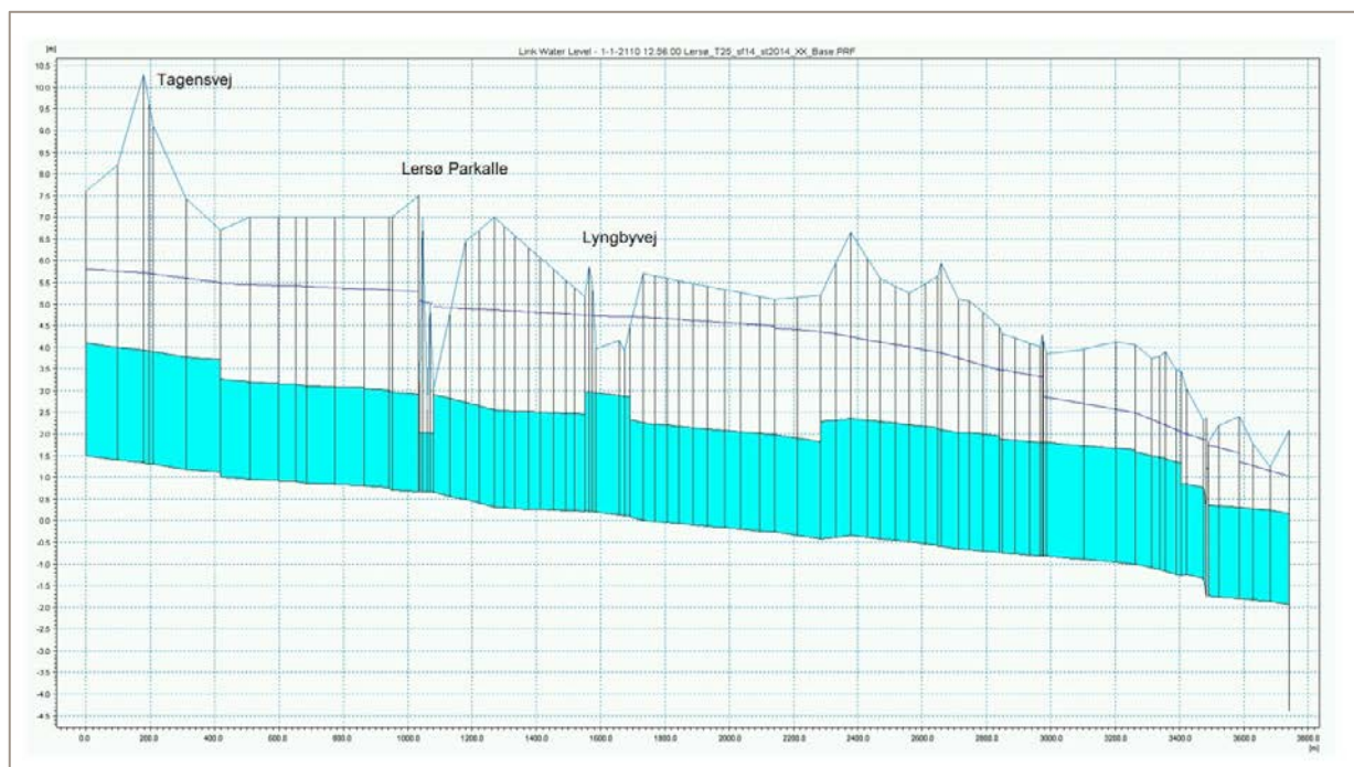
Figur 4-6 Længdeprofil af Lersøledningen og Vilhelmsdalsløbet fra Lygten til udløbet i Svanemøllebugten med stuvningsniveau for 25 års regnhændelse i 2010. Sø- vand fra Emdrup Sø ledes til stuvningsbassin øst for Lyngbyvej ved Ryparken.
