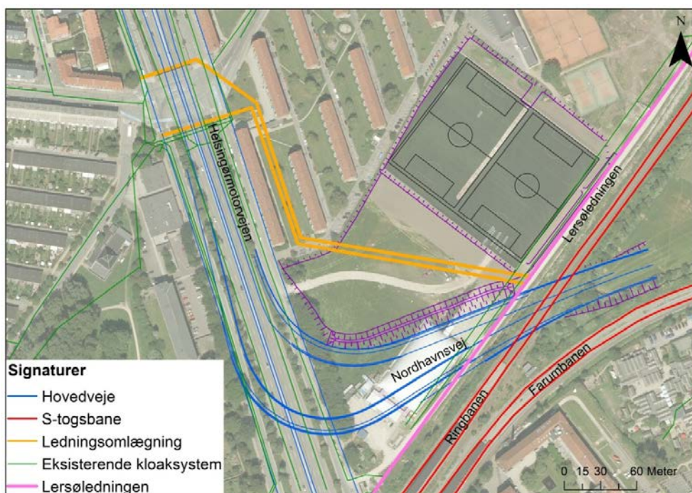
Figur 5-6 Planlagt omlægning af overløbs- og søvandsledninger ved Lyngbyvej fra vest- til østsiden af Helsingørsmotorvejen. De brune ledninger på arealet mellem boldbanerne og vejanlæggene viser omlægningen.
