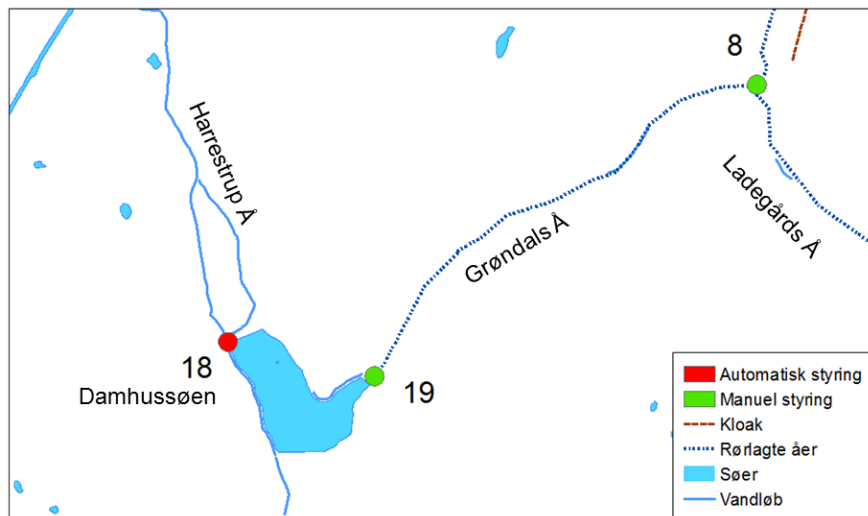
Figur 25 Kort over det vestlige vandområde og styrestrategiens reguleringspunkter. Rød indikerer lokalitet med automatisk styring og grøn med manuel styring. Tallene henviser til listen på side 8.
