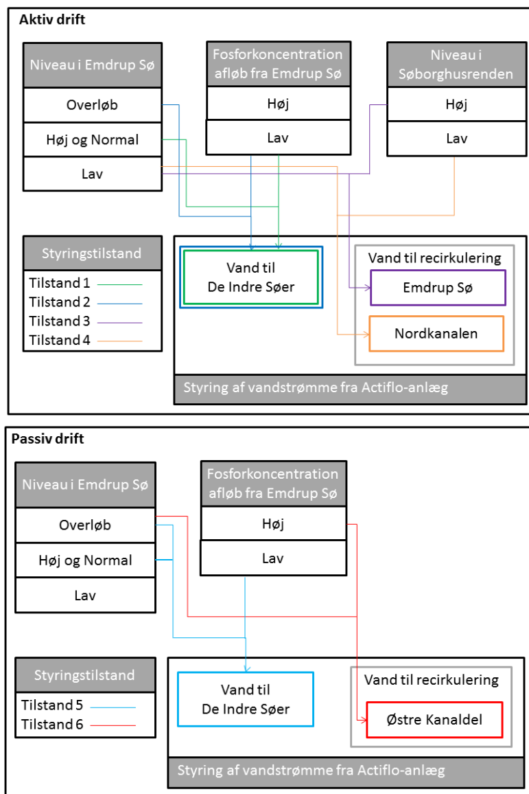
Figur 13 Skematisk illustration af styringstilstandene for de automatiske styring af Actiflo®-anlægget og vandstrømmene omkring Emdrup Sø for aktiv og passiv drift af Actiflo®-anlægget.
