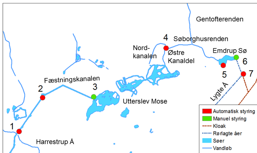
Figur 7 Kort over det nordlige vandområde og styrestrategiens reguleringsskemaer. Rød indikerer lokalitet med automatisk styring og grøn med manuel styring. Tallene henviser til listen på side 8.
