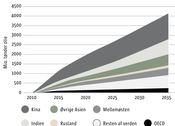
FIGUR 3 // Væksten i udviklingslandene vil føre til en 33 pct. stigning i energiforbruget frem mod 2035 – selv hvis de nuværende klimamålsætninger på nationalt niveau gennemføres. Kilde: IEA, World energy outlook 2012 .
